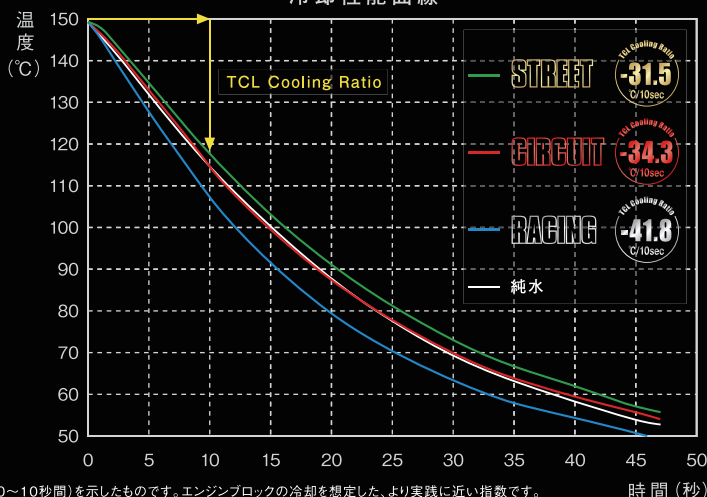
冷却性能曲線
